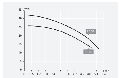
Curvas características
