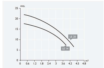
Curvas características
